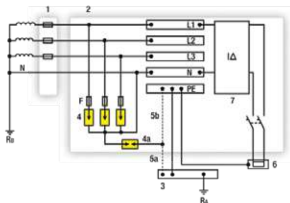
Installazione di SPD in un sistema TT con interruttore differenziale a valle
